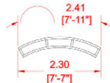
Vista Superior de una sección
