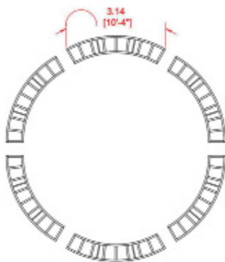
Vista Superior (6 secciones)
