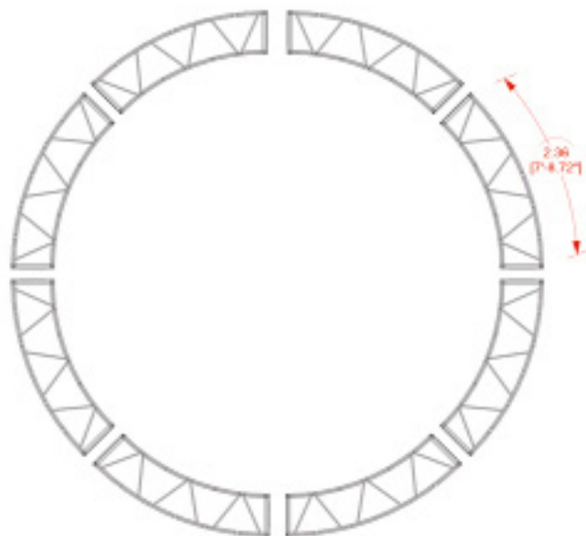
Vista superior 8 secciones
