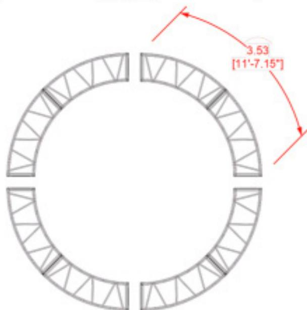
Vista superior 4 secciones
