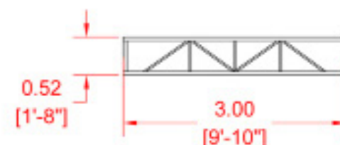
Vista Frontal de una sección
