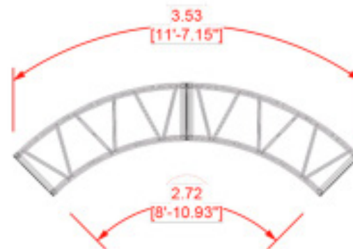
Vista superior de una sección
