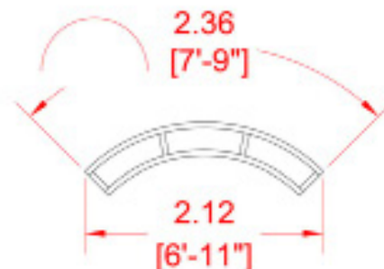
Vista Superior de una sección
