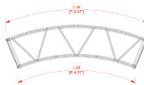
Vista superior de una sección
