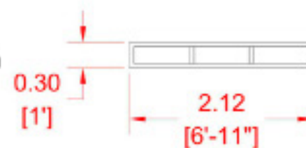
Vista Frontal de una sección
