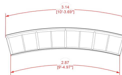
Vista superior de una sección
